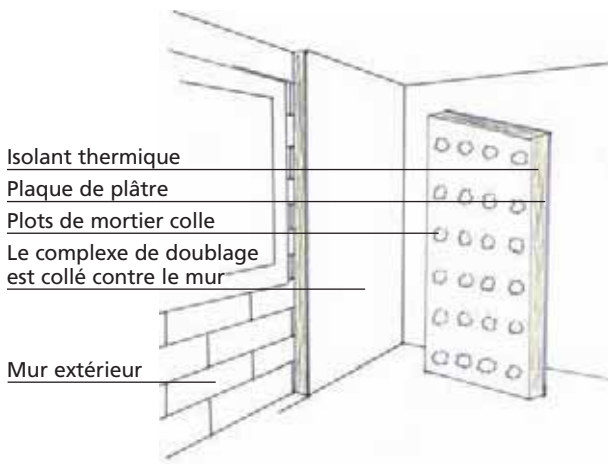
Isolation par l'intérieur par complexe collé
