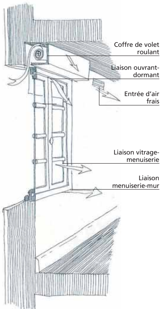
Passage d'air à travers une façade
