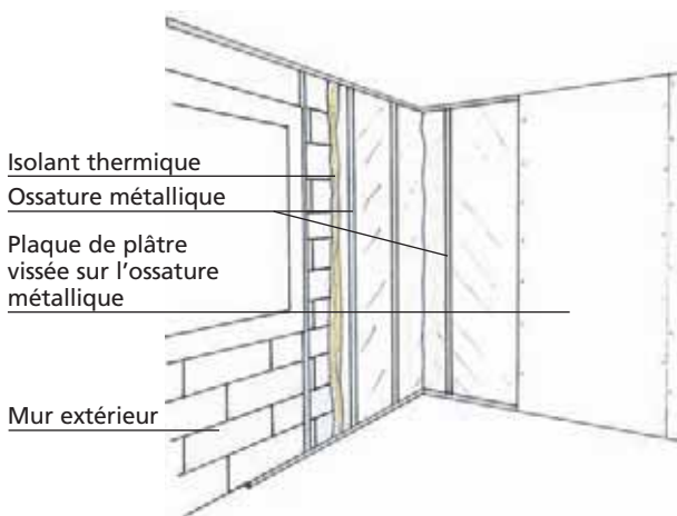
Isolation par l'intérieur par doublage sur ossature
