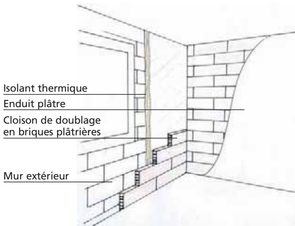
Isolation par l'intérieur par doublage maçonné
